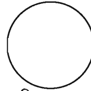
চিত্র-১: বৃত্ত
