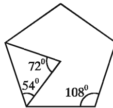
সুখম পঞ্চভুজ
