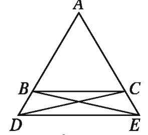
চিত্র ২
