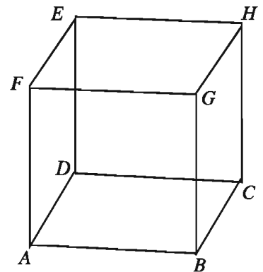
ঘনক
