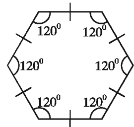
সুখম ষড়ভুজ
