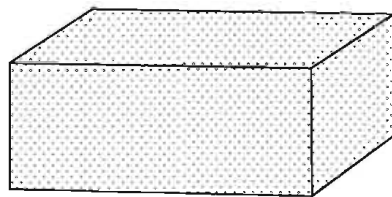
আয়তাকার ঘনবস্তু
