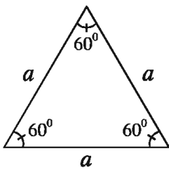
সমবাহু ত্রিভুজ
