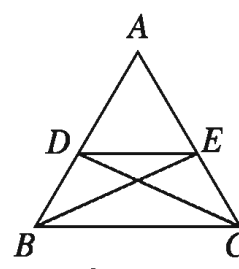
চিত্র ১
