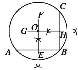
চিত্র-১: বৃত্ত
