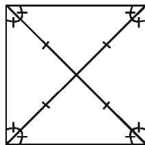
বর্গক্ষেত্র
